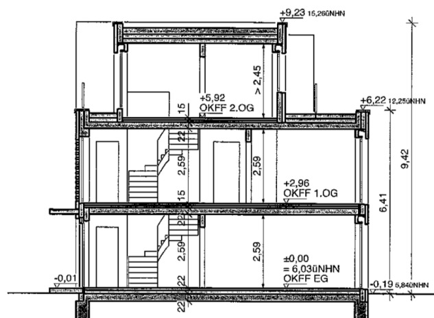
Schnitte
