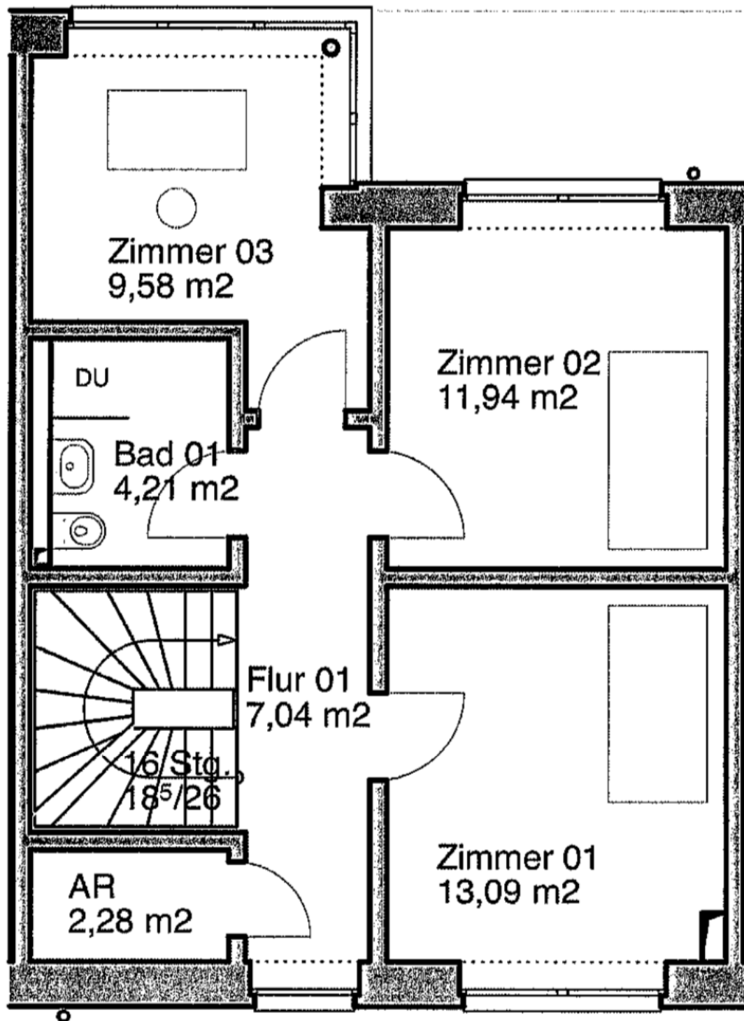
Grundrisse
